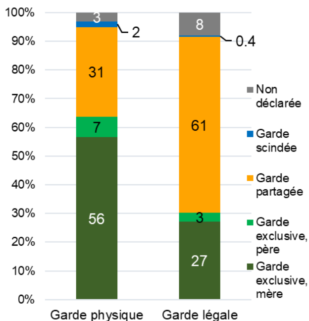
Graphique 1 La garde dans les ordonnances de six cours supérieures, 2018-2019
