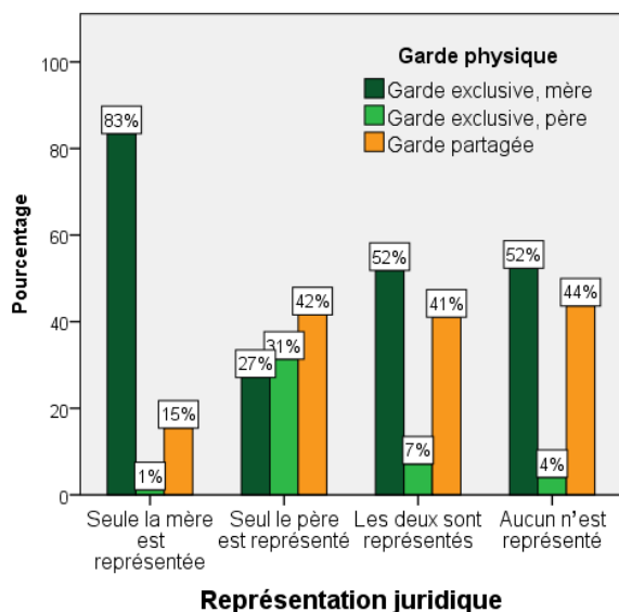
Graphique 3 - Représentation juridique et garde physique dans six cours supérieures, 2018-2019
